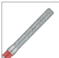
#2110F Grain Fin Cylindre Ø1.4x8mm
