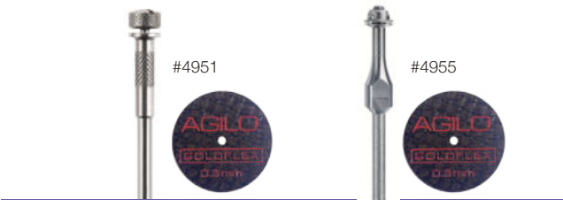
Mandrins à changement rapide pour disques Schnellspann Scheibenhalter Quick-change mandrels for discs Tige/Schaft/Shank Ø2.34mm-3/32"
